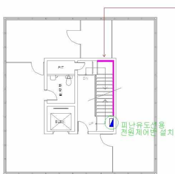
구.관제탑 7층 평면도
