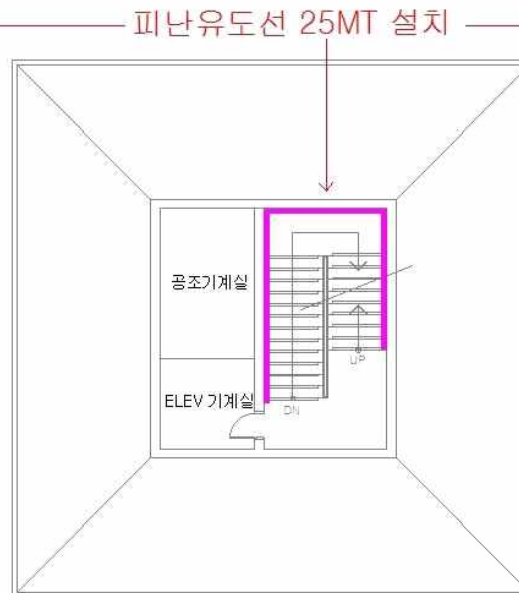
○ 구.관제탑 8층 평면도 축척 = 1/100
