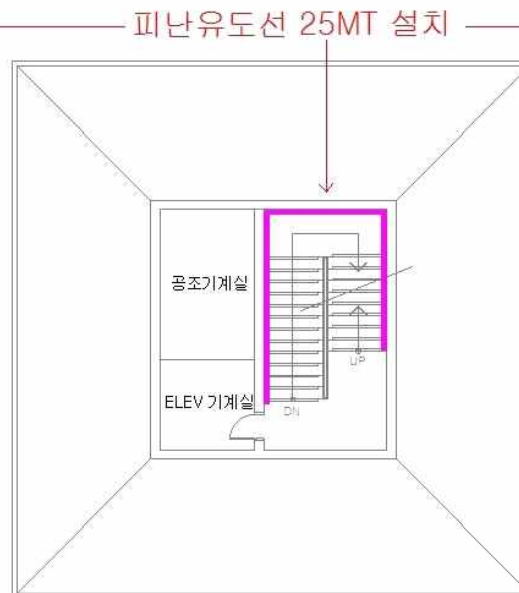
구.관제탑 8층 평면도
